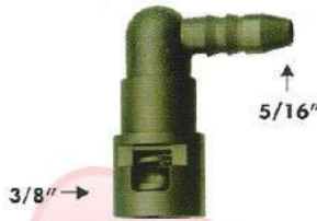
459 051 engate rápido pop top Ø 3/8x5/16" 90°
