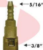
459 046 engate rápido pop top Ø 5/16" reto
