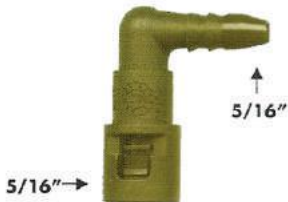
459 048 engate rápido pop top Ø 5/16" 90°
